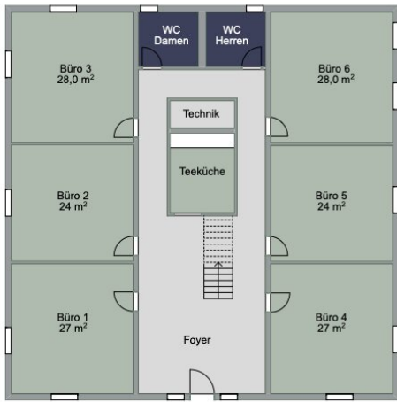
ERDGESCHOSS
