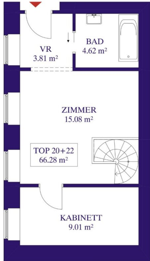
1. GESCHOSS
