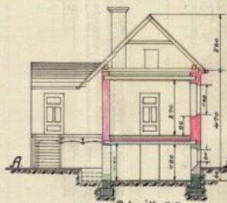
Schnitt A-B
