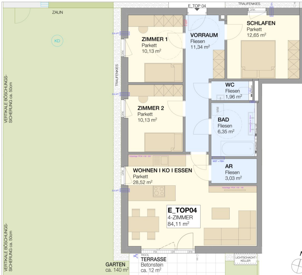
LAGE IM GESCHOSS ERDGESCHOSS
