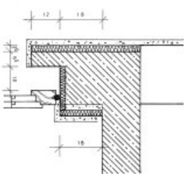
STURZAUSSCHÜTTUNG M 1/1.5
