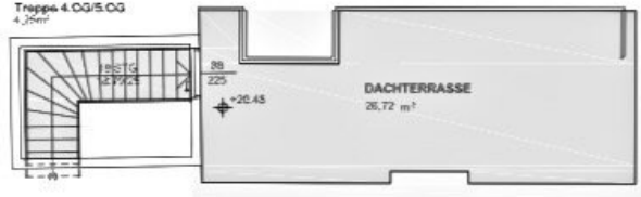
Grundriss 5. Dachterrasse
