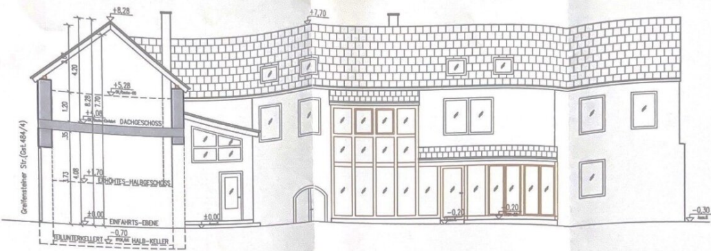
SÜDANSICHT
