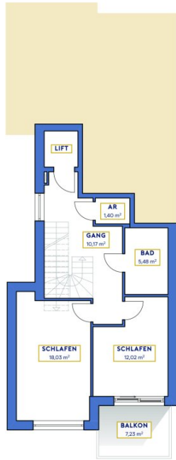
OBERGESCHOSS M 1:100
