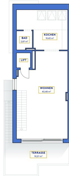
DACHGESCHOSS 1:100
