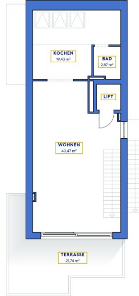
DACHGESCHOSS 1:100
