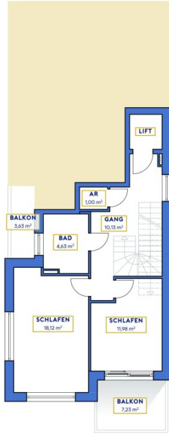
OBERGESCHOSS M 1:100
