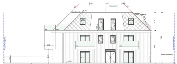
ANSICHT SÜD
