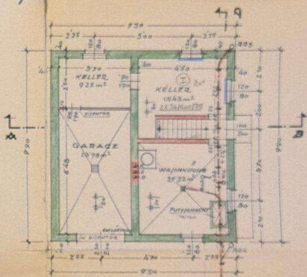
KELLERGESCHOSS
