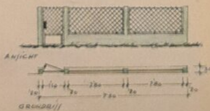
EINFRIEDUNG
