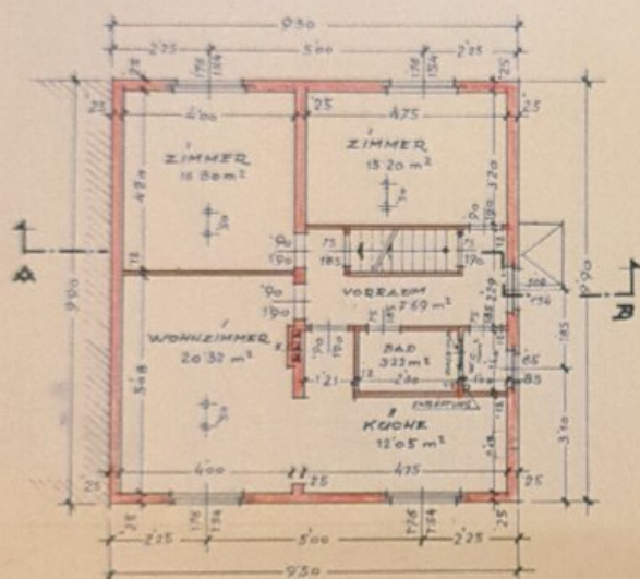
ERDGESCHOSS
