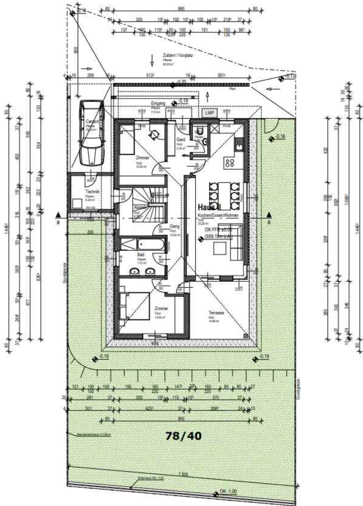
Erdgeschoss M.1:100 Nettofläche + Technik: 97,69 m²
