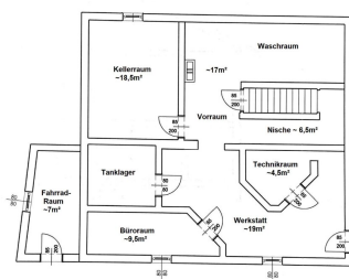
Skizze Grundriss Kellergeschoss
