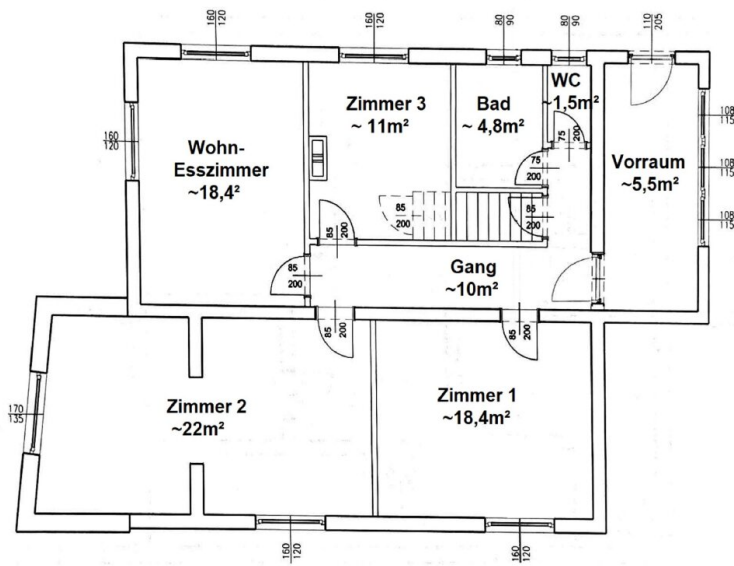
Skizze Grundriss Erdgeschoss
