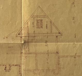
SCHNITT A-B
