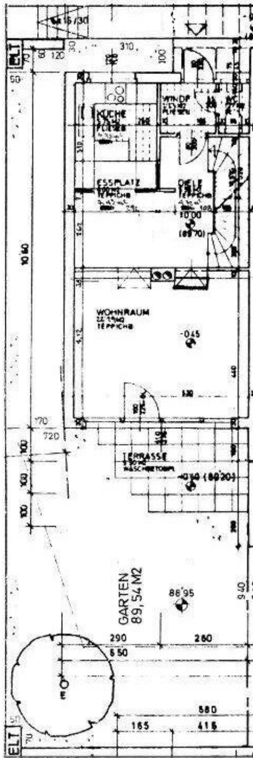
ERDGESCHOSS
