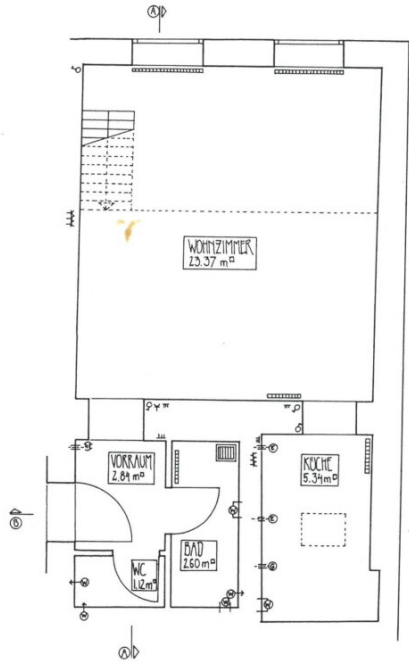
ERDGESCHOSS
