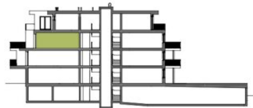
LAGE GESCHOSS
