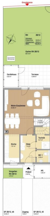
ERDGESCHOSS
