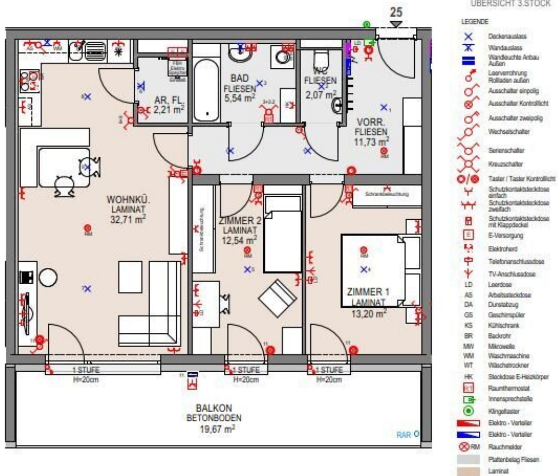
ÜBERSICHT 3.STOCK
