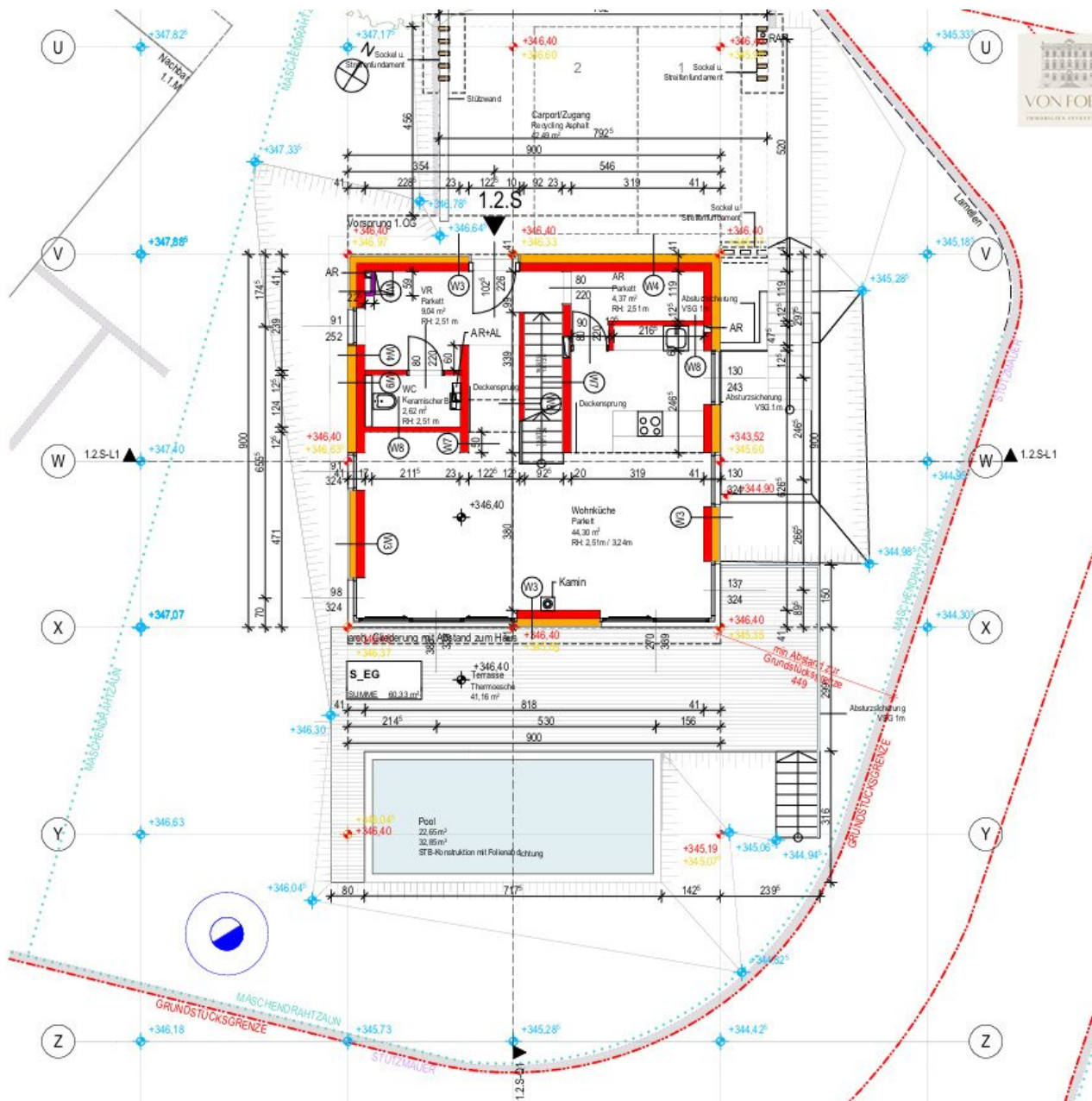
Grundriss 1.2.S-EG
