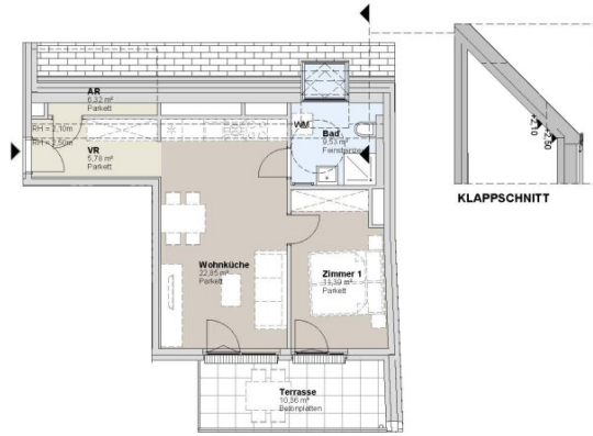
2. DACHGESCHOSS STRASSENBAUKÖRPER
