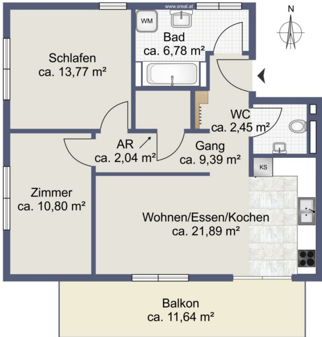
Skizze 1.Obergeschoss
