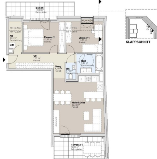
1. DACHGESCHOSS STRASSENBAUKÖRPER
