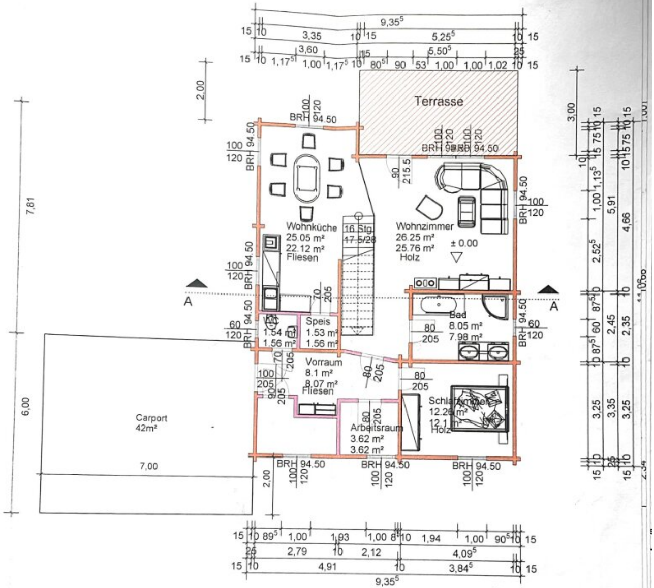
Erdgeschoß
