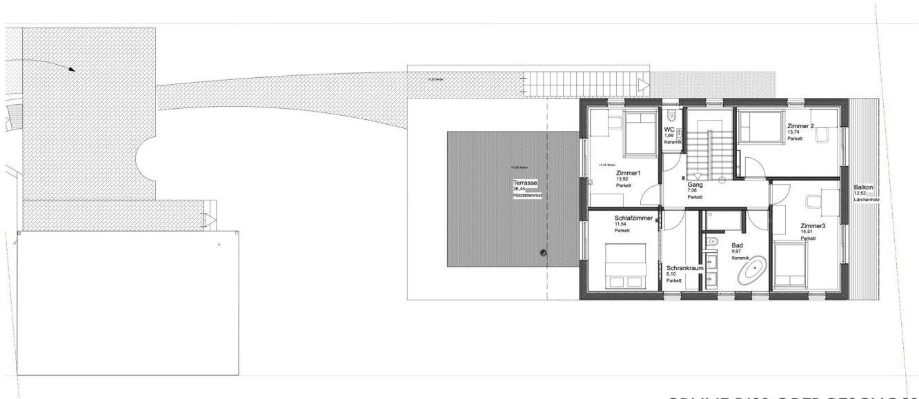
GRUNDRISS OBERGESCHOSS
