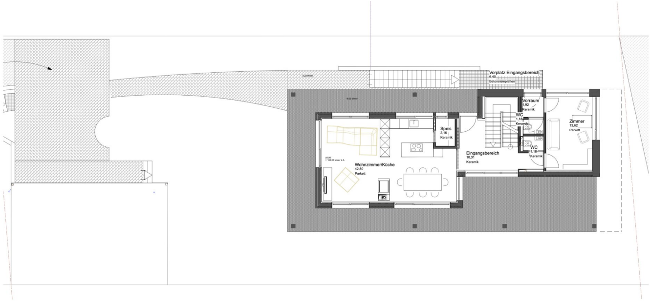
GRUNDRISS ERDGESCHOSS
