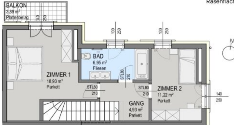
GRUNDRISS: ERDGESCHOSS
