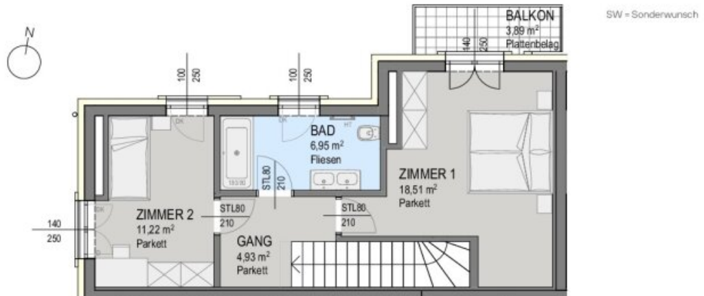
GRUNDRISS: ERDGESCHOSS
