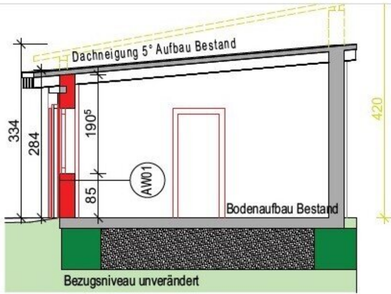
SCHNITT - A
