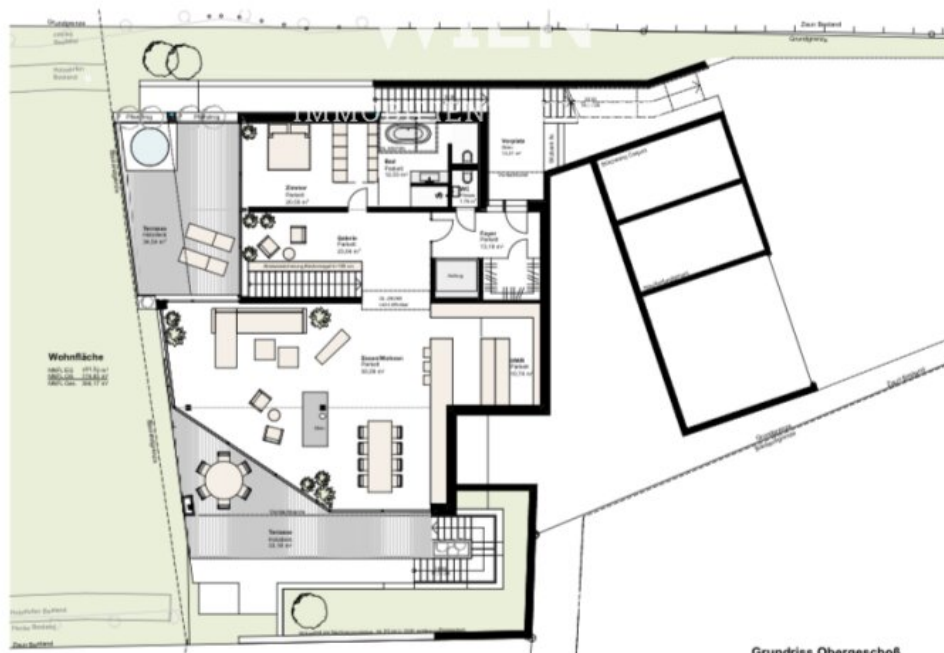
Grundriss Obergeschoß Villa Heiligengestade
