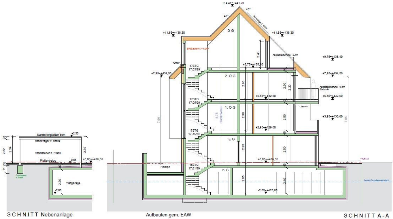
SCHNITT Nebenanlage
