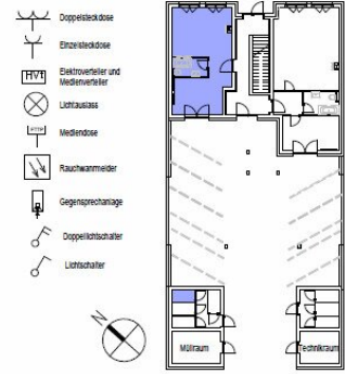
Erdgeschoss Vorderhaus
