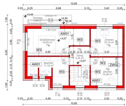
GRUNDRISS OBERGESCHOSS 1:100
