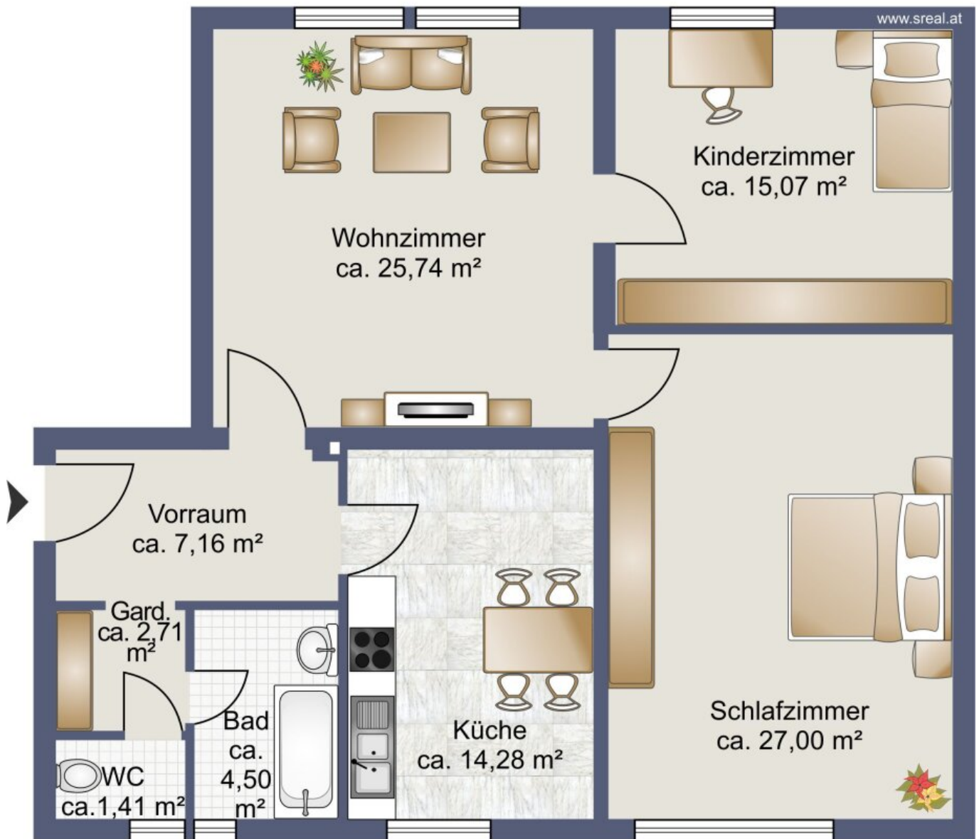
Skizze Wohnung
