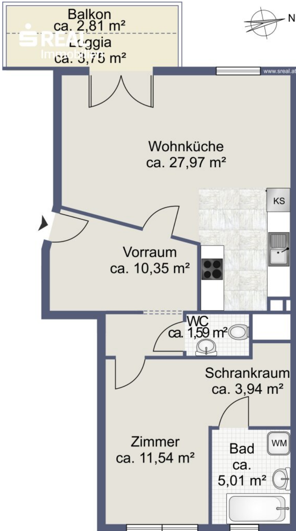
Skizze Wohnung
