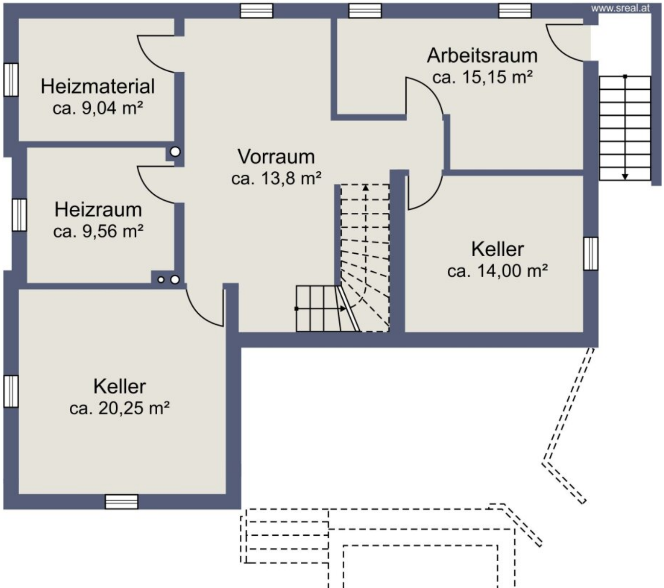
Skizze Kellergeschoss
