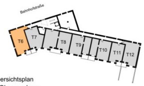
Übersichtspl 1. Obergeschoss
