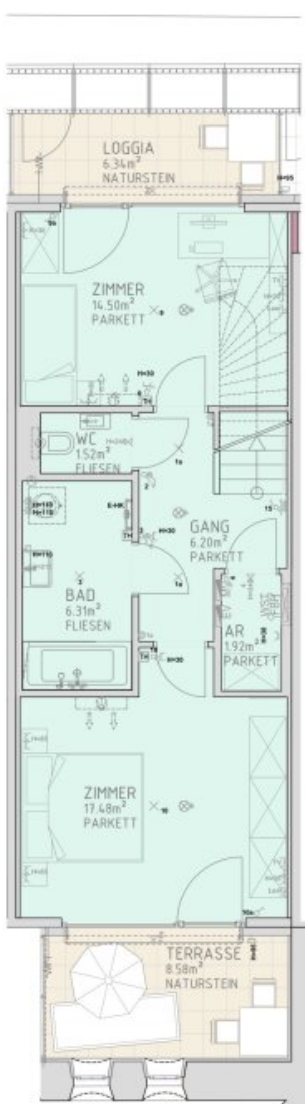
1.DACHGESCHOSS M 1:50
