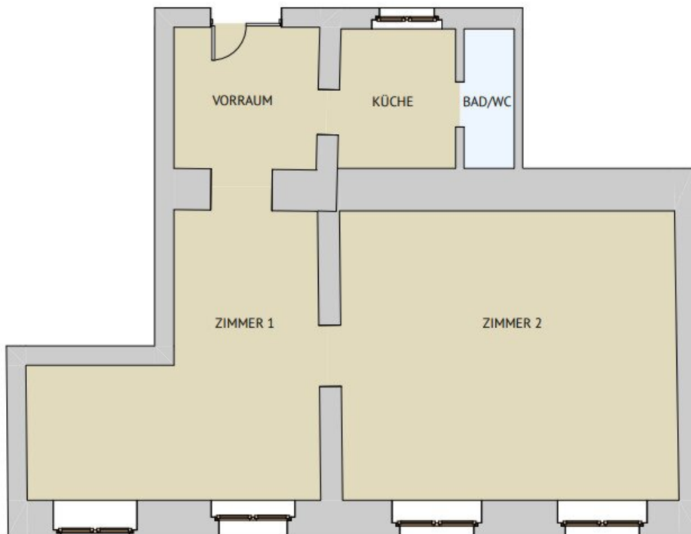
GRUNDRISS M 1:100
