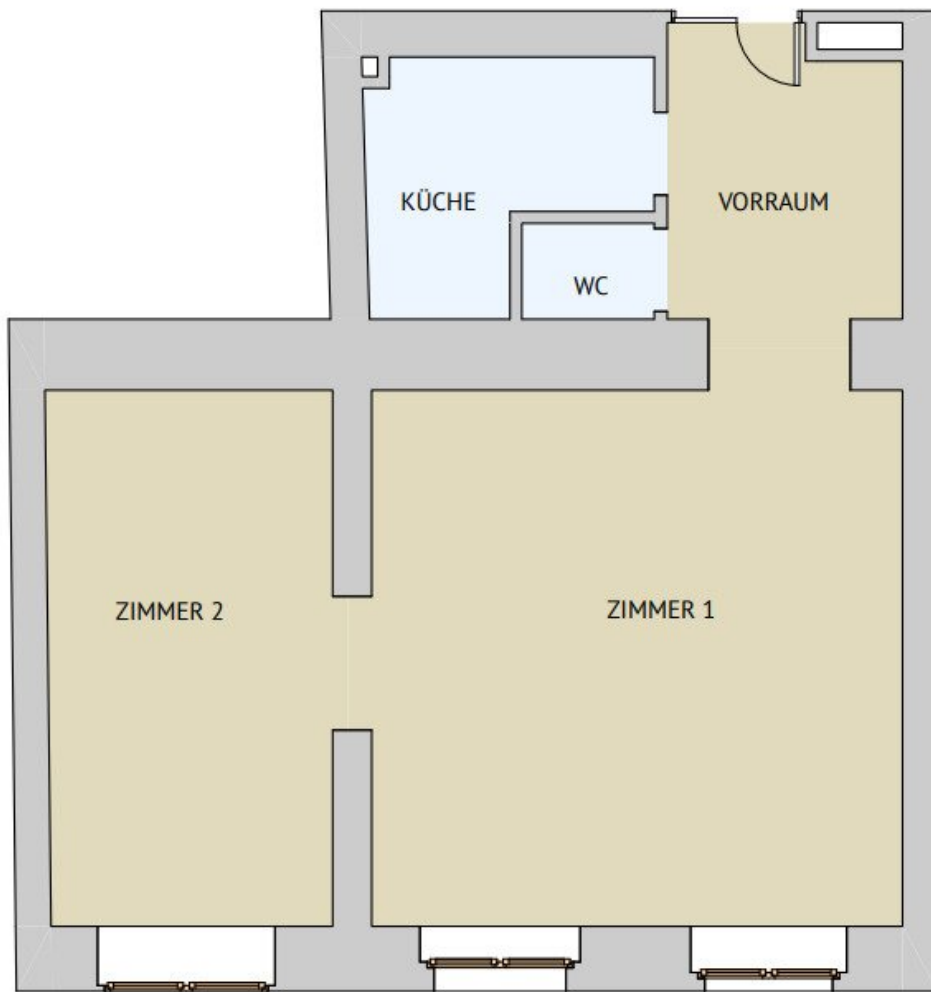
GRUNDRISS M 1:100
