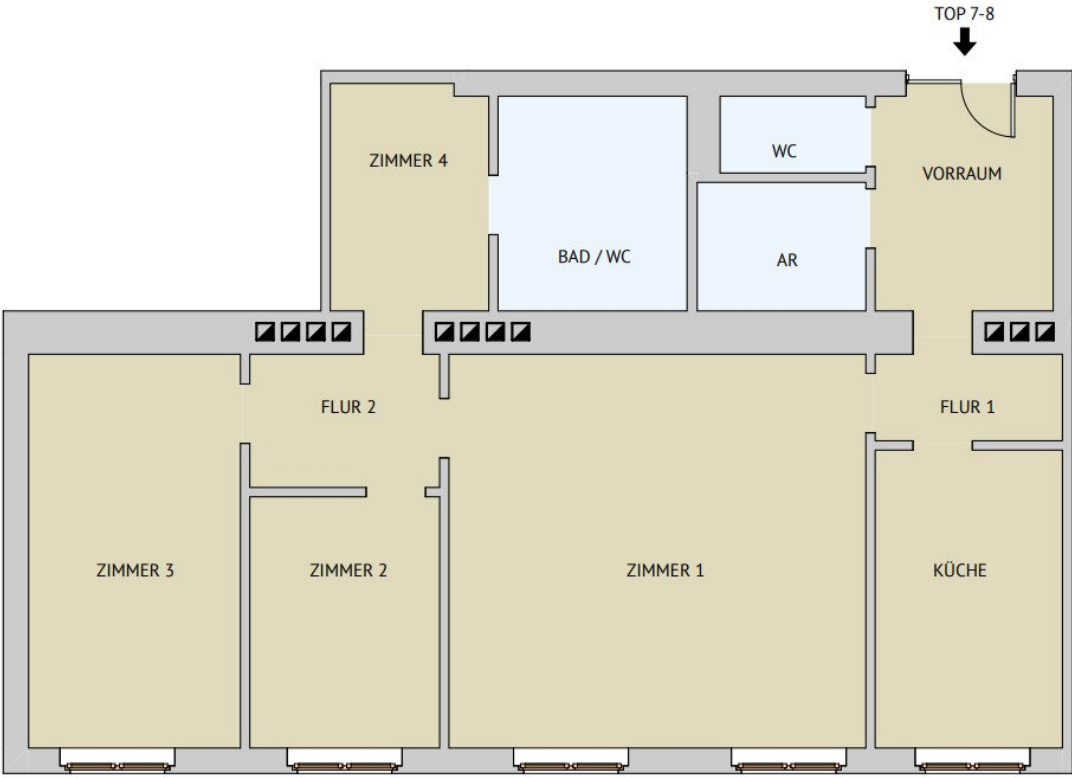
GRUNDRISS M 1:100
