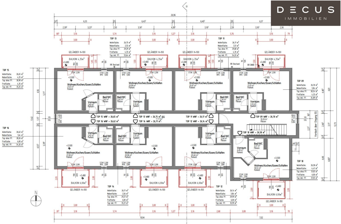
REGELGESCHOSS 1-3 M 1:100
