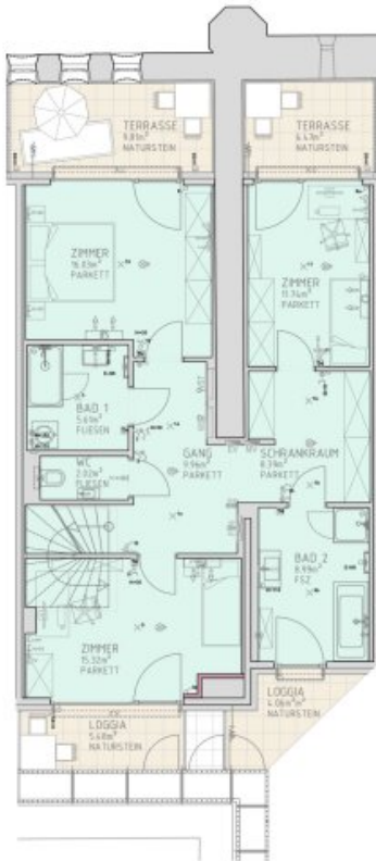
1.DACHGESCHOSS M 1:75
