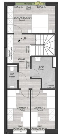
1. OG
