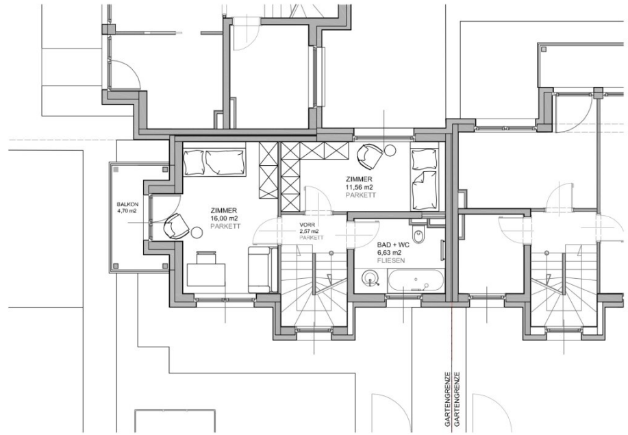
OBERGESCHOSS
