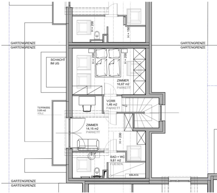
DACHGESCHOSS
