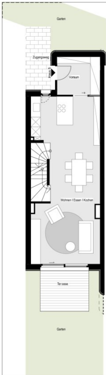
Erdgeschoß
