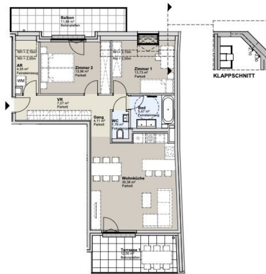
1. DACHGESCHOSS STRASSENBAUKÖRPER
