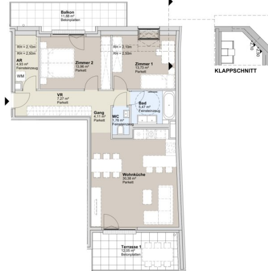
1. DACHGESCHOSS STRASSENBAUKÖRPER
