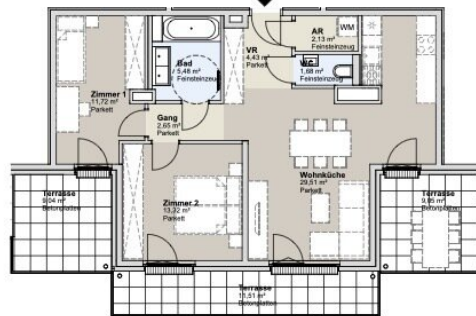
2. DACHGESCHOSS STRASSENBAUKÖRPER
