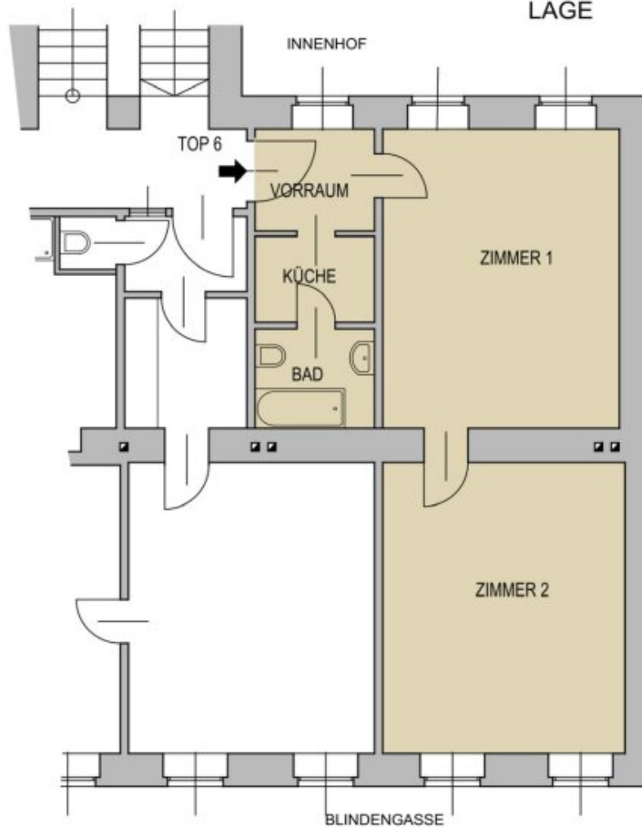
GRUNDRISS M 1:100
