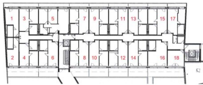
1. OBERGESCHOSS M 1 : 200
